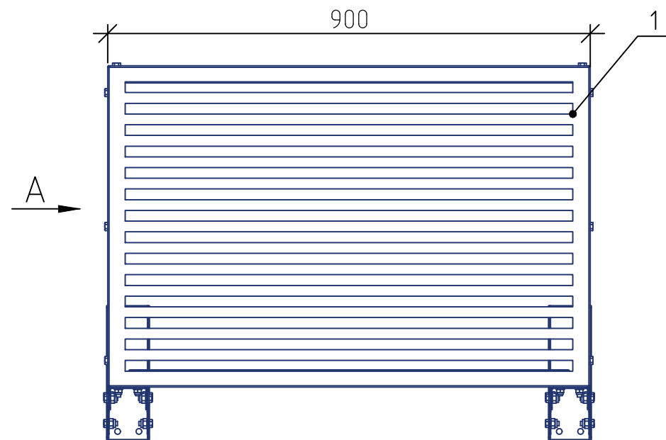
Корзина для кондиционера KORZ.600(h)x900x550.T1
